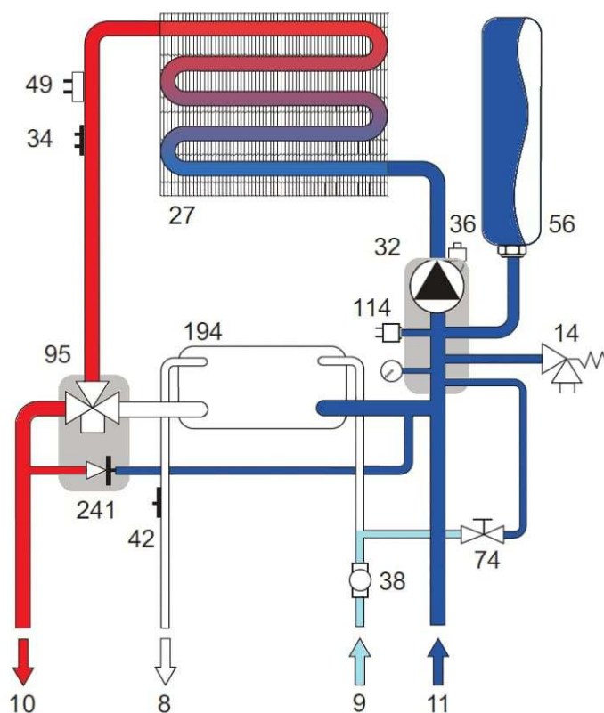
рис. 17 – Отопительный контур
