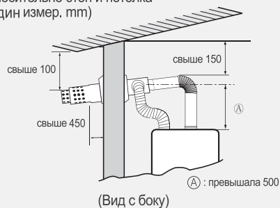
· Расположение дымохода относительно стен и потолка (Един измер. mm)
