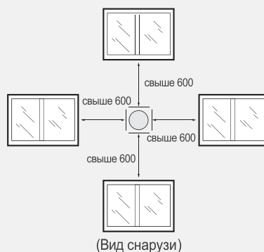
· Расположение конца дымохода по отношению к окнам
